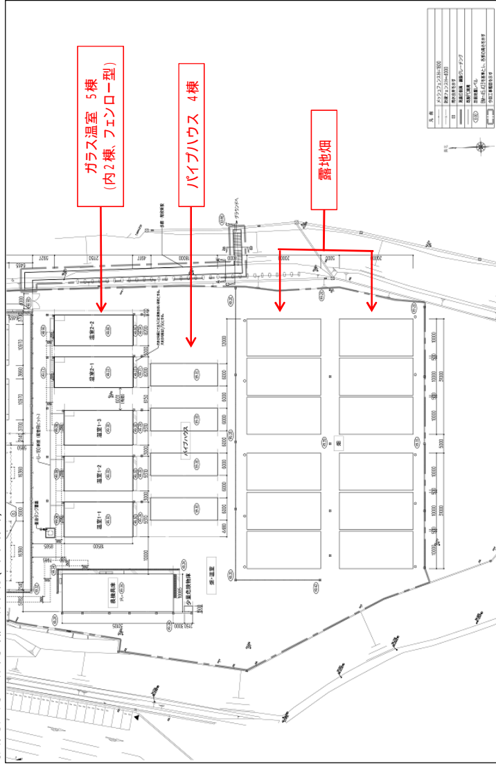
摂南大学 農学部 農場 (平面図)
